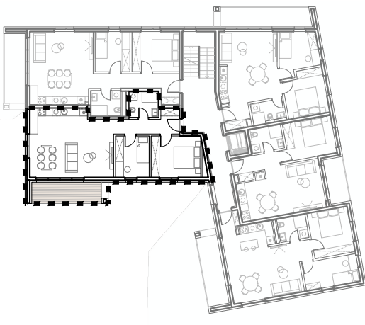
POZICIJA STANA 10 NA TLOCRTU 1. KATA
