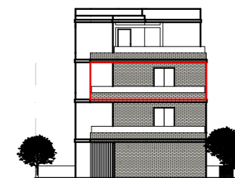
SJEVERNO PROČELJE
