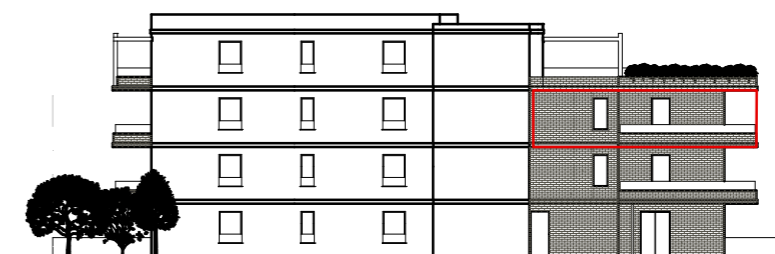
ISTOČNO PROČELJE
