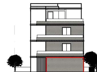
SJEVERNO PROČELJE
