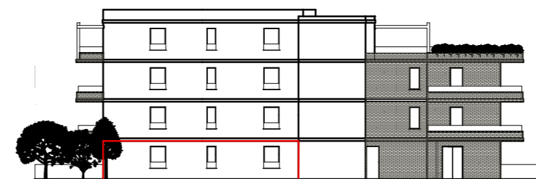
ZAPADNO PROČELJE
